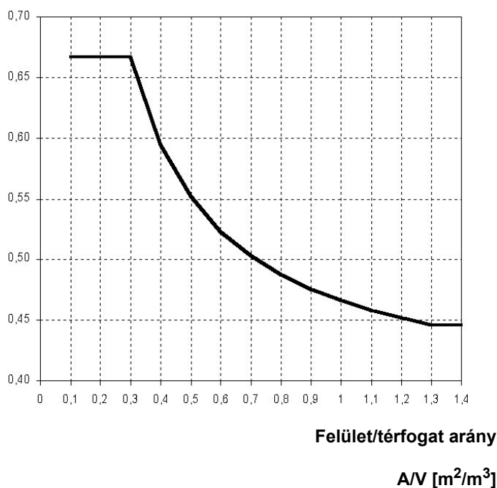
2. ábra: Az átlagos hőátbocsátási tényező követelményértékei
