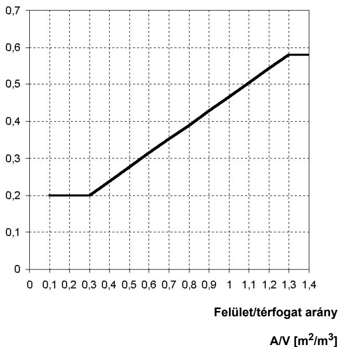
1. ábra: A fajlagos hővesztégtényező követelményértéke
